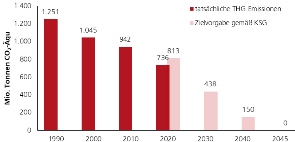
Abbildung 2 | Treibhausgas-Emissionen in Deutschland seit 1990 und Treibhausgas-Minderungsziele gemäß Bundes-Klimaschutzgesetz (KSG) (target GmbH nach [10])
